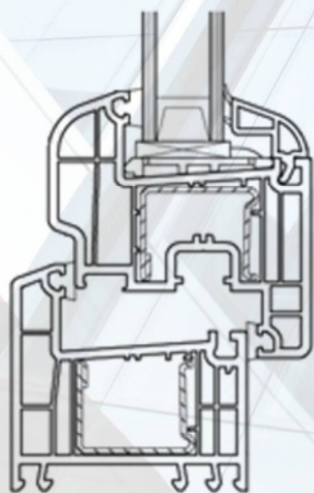
Zespolenie 2-szybowe
