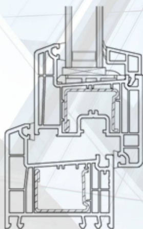
Zespolenie 2-szybowe
