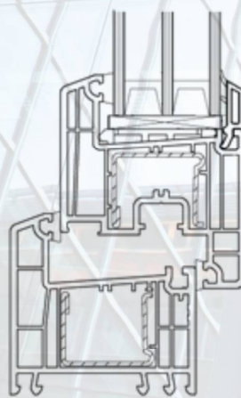
Zespolenie 3-szybowe
